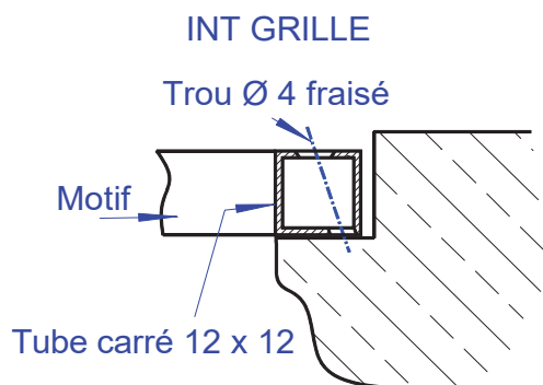
Fixation type 1 (prix du tarif)
