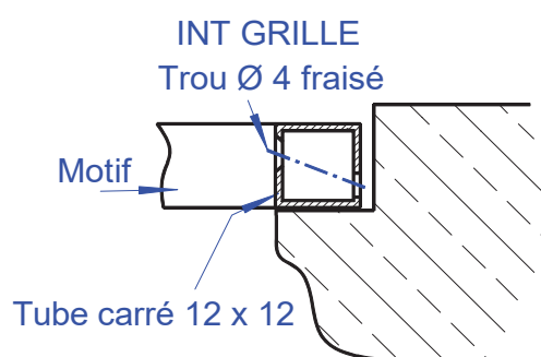
Fixation type 3 (prix du tarif)
