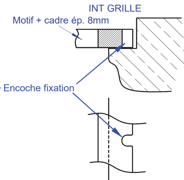
Fixation type laser (prix du tarif)
