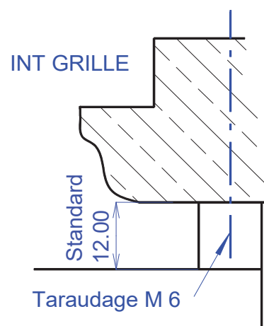
Fixation type 4 (option applique)
