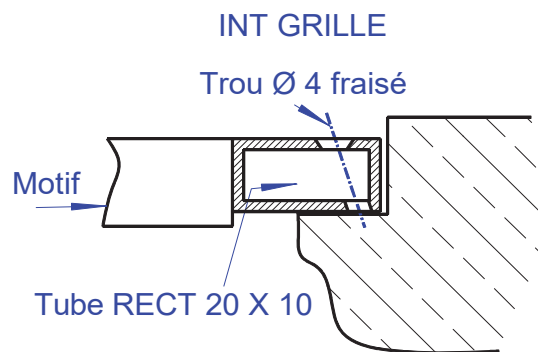
Fixation type 2 (prix du tarif)
